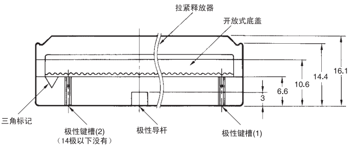
尺寸表
