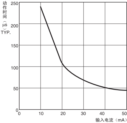
G3DZ-1R5PLG
