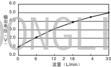
D6F-05N7-000
