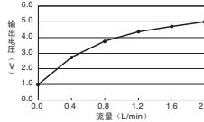
D6F-02L7-000
