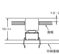
参考尺寸
