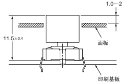
参考尺寸
