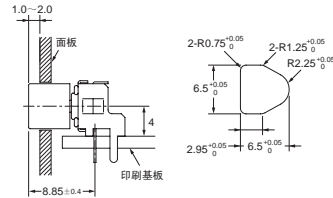
面板切割尺寸
