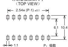
印刷基板加工尺寸 (TOP VIEW)
