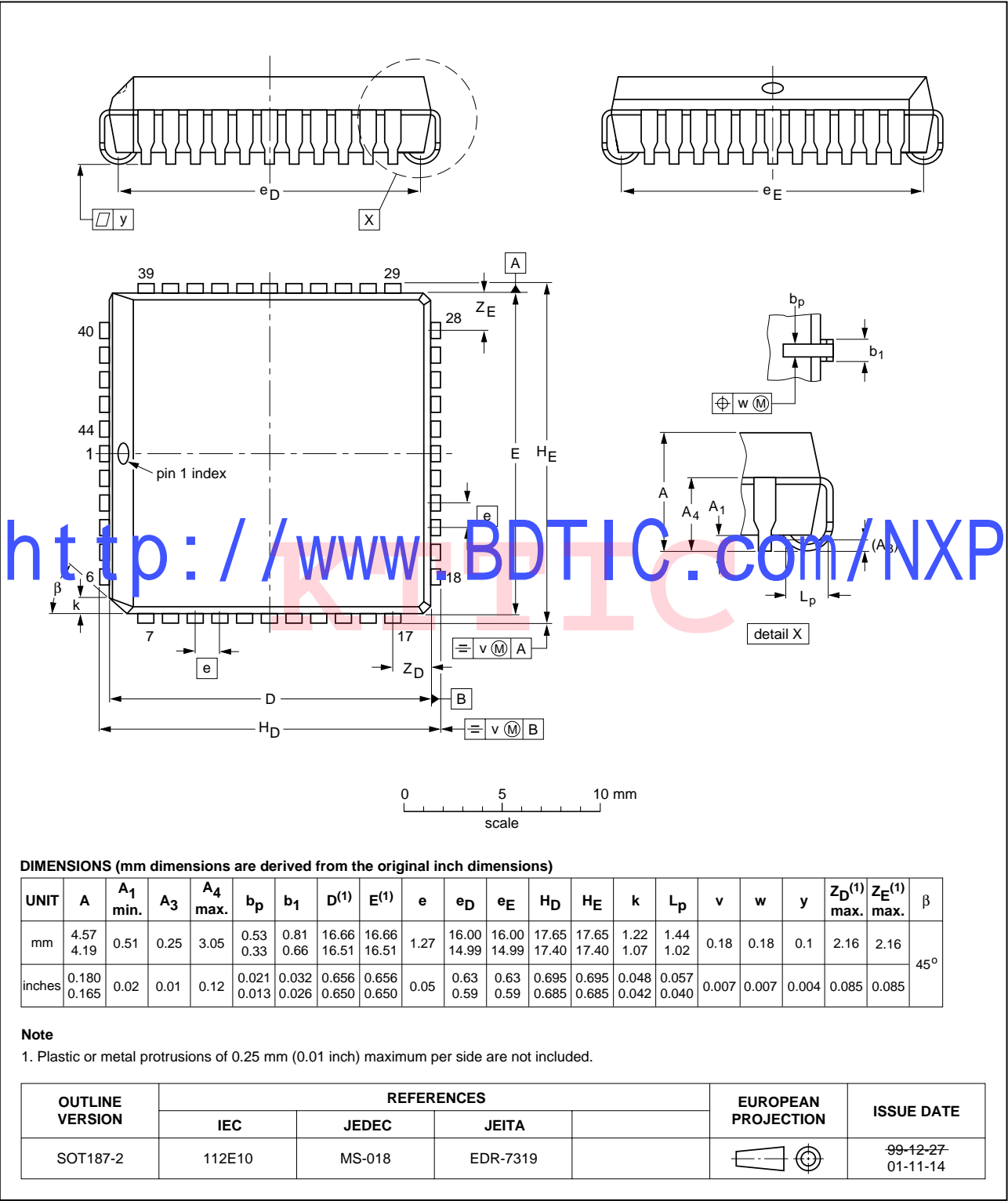
Fig 22. PLCC44 (SOT187-2).
