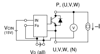
Fig. 2 V_{ce} Test
