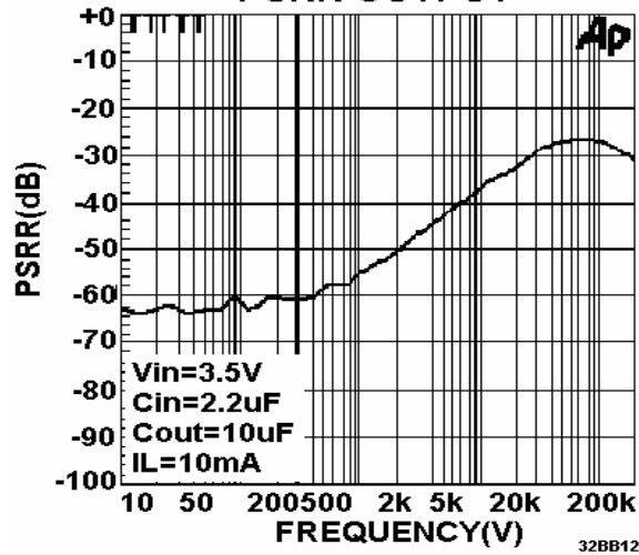
PSRR OUTPUT
