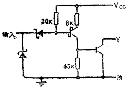
参考线路(1/6)
